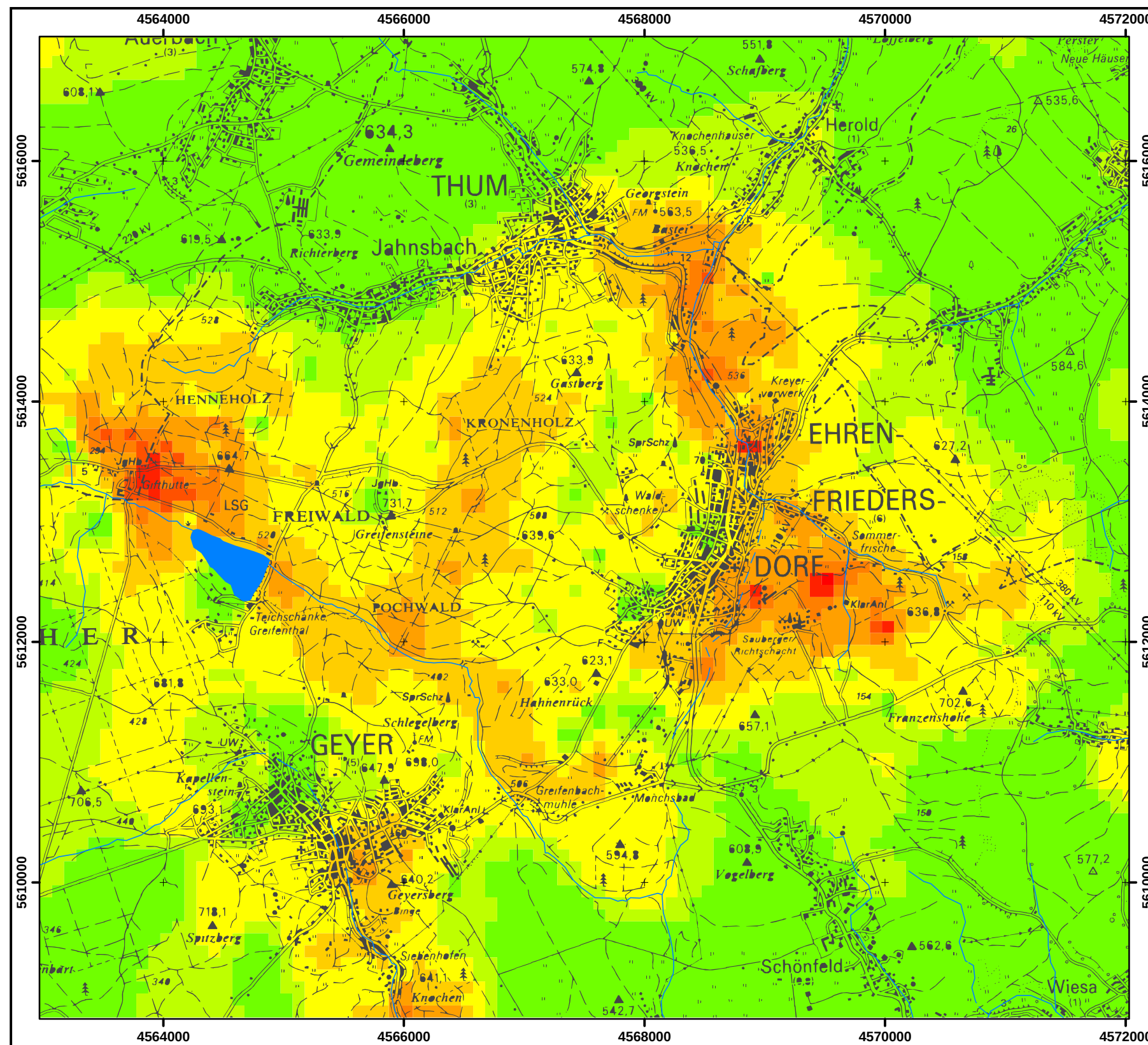
Abb. 7: Arsen im mineralischen Oberboden
