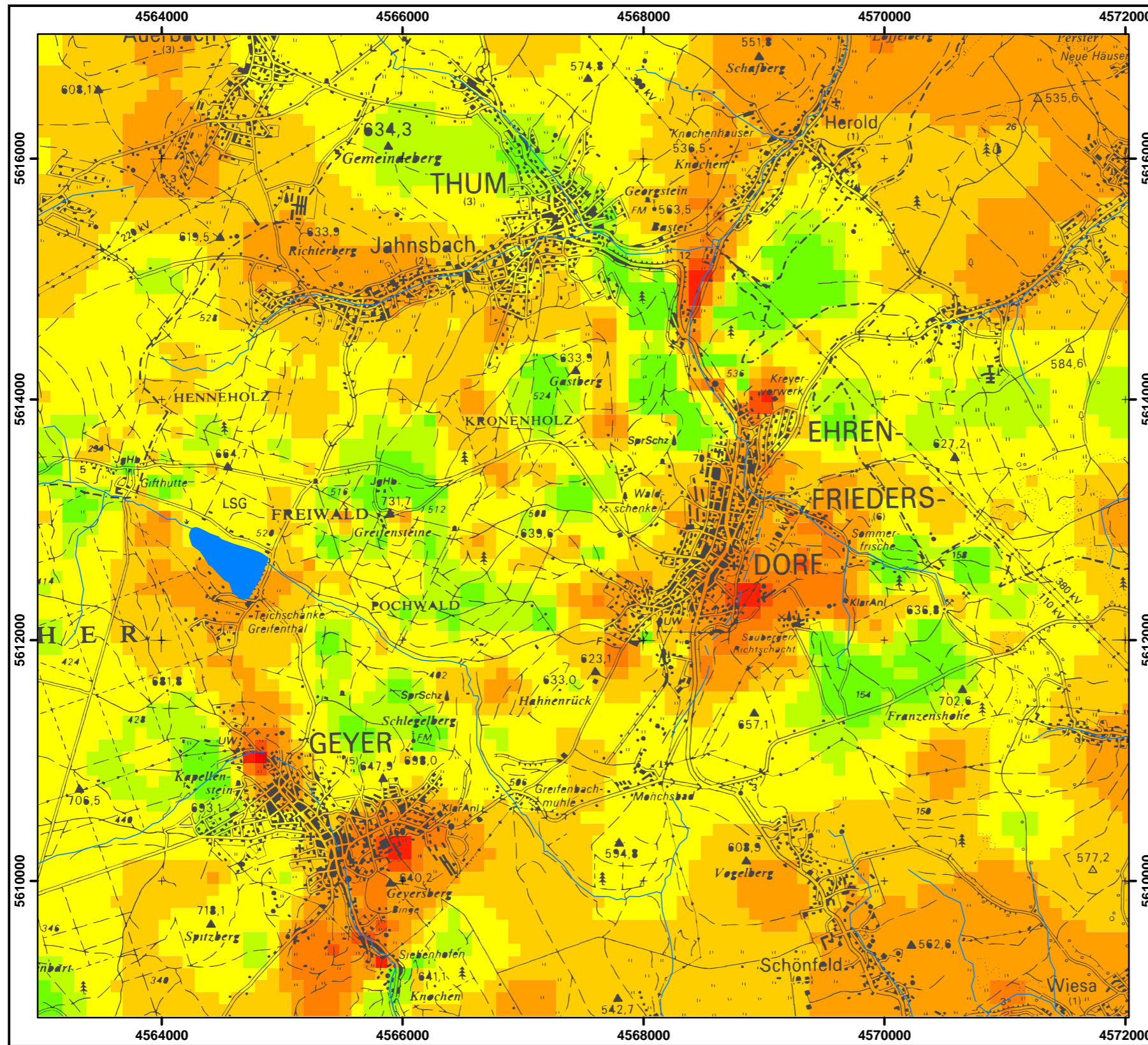
Abb. 25: Cadmium im Unterboden
